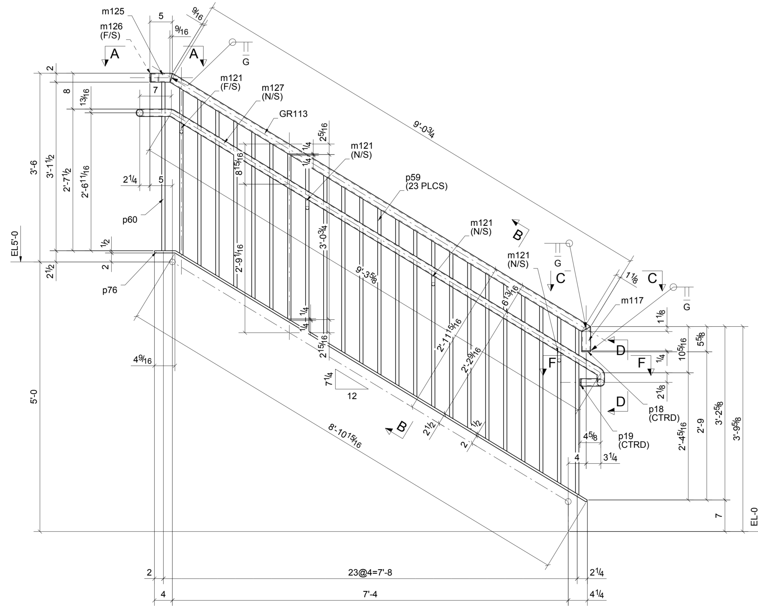
1 - GUARDRAIL -GR113
